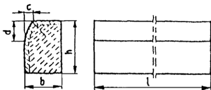
Rys. 1. Wymiarowanie krawężników
