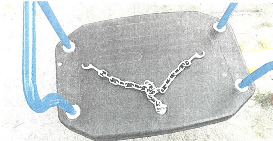
Fot. nr 6. KARUZELA KRZYŻOWA - karabińczyki do wymiany
