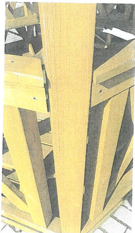
Fot. nr 5. WIATA DREWNIANA - mocowanie poręczy do poprawy
