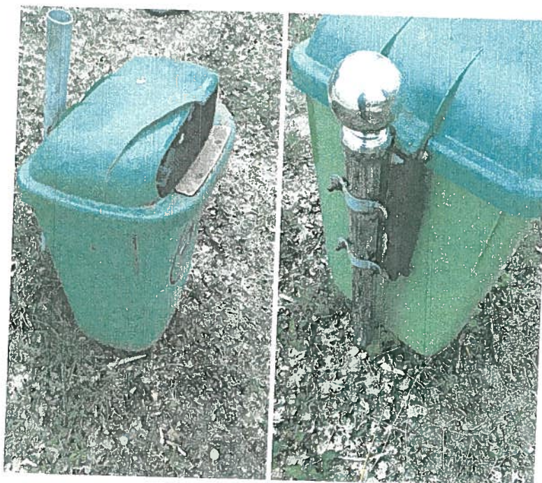
Fot. nr 3, 4, 5, 6. KOSZ NA ŚMIECI PLASTIKOWY: umyć pokrywę (1 szt.), pokrywa uszkodzona do wymiany (1 szt.), pokrywa uszkodzona i mocowanie pojemnika uszkodzone do wymiany (1 szt.), pokrywa kosza uszkodzona do wymiany, mocowanie pojemnika oczyścić z rdzy, zabezpieczyć antykorozyjnie i pomalować (1 szt.).
